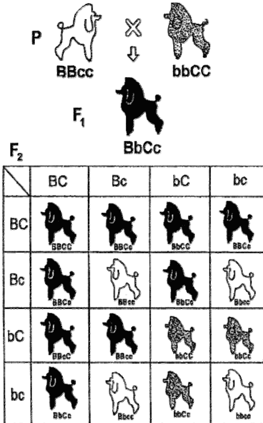
Рис. 19. Схема дигибридного расщепления с рецессивным эпистазом: во F 2 получено 9 черных: 3 коричневых: 4 белых собаки.
